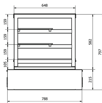
VISTA LATERAL
