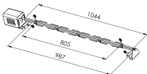
Dimensiones del Spiedo
