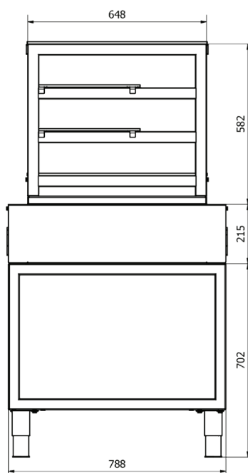
VISTA LATERAL
