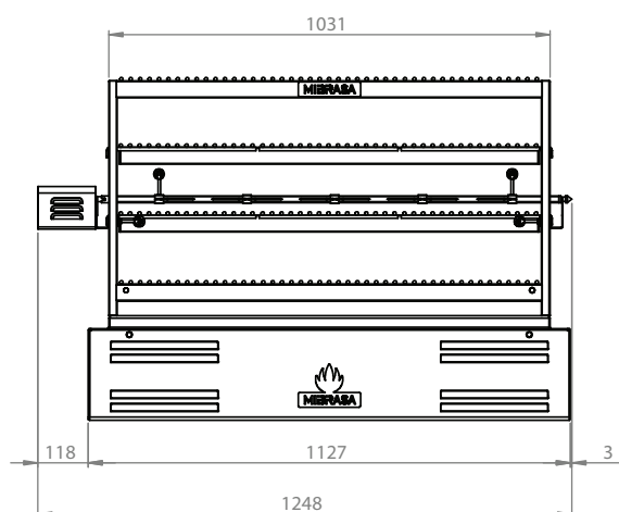
Vista frontal montado
