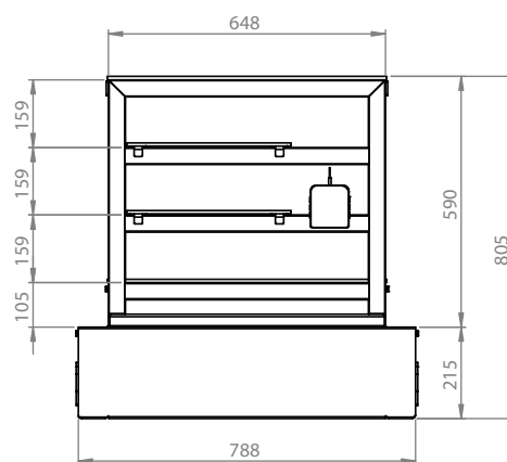
Vista lateral montado
