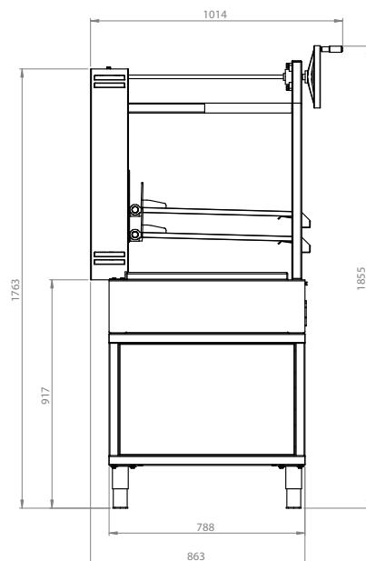
VISTA LATERAL
