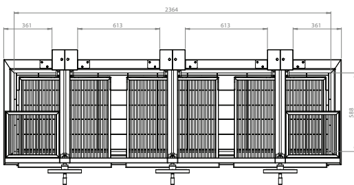
VISTA SUPERIOR
