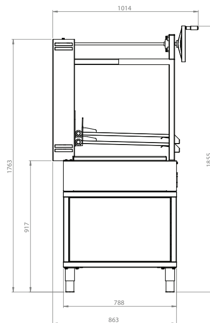
VISTA LATERAL
