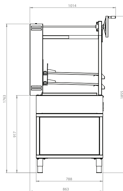
VISTA LATERAL
