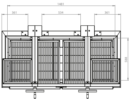
VISTA SUPERIOR
