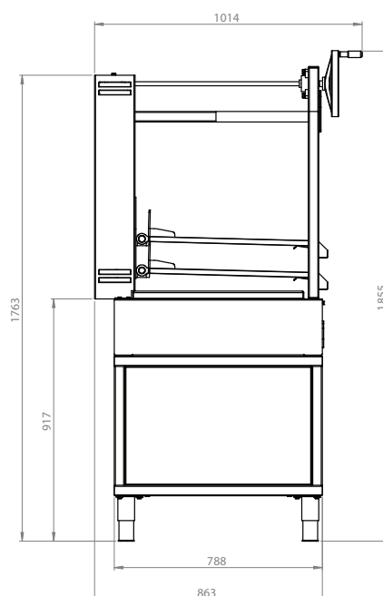
VISTA LATERAL
